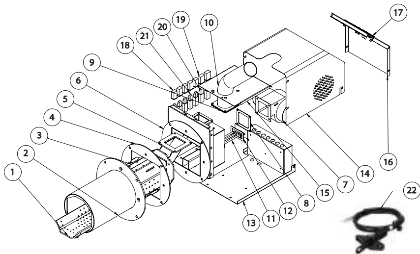
10. Ábra. Pellet égőfej alkatrészek Pell Eco
