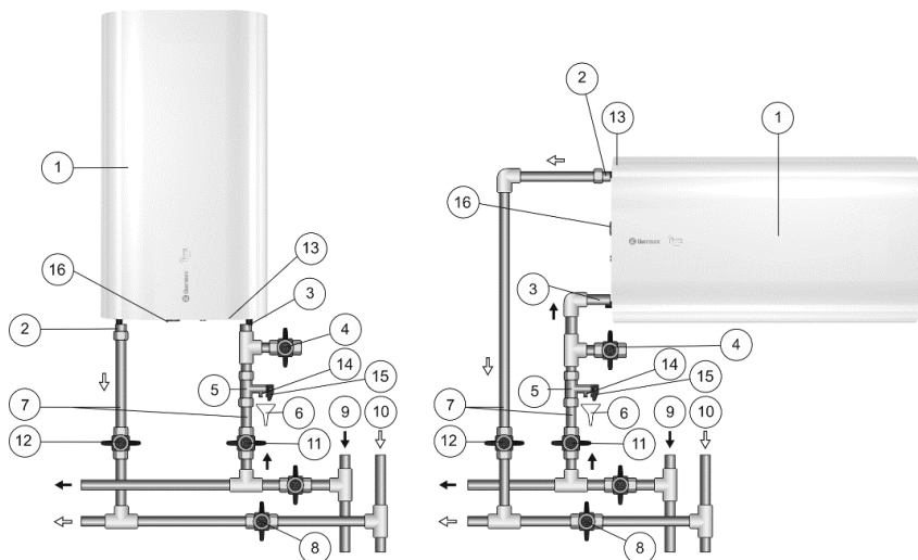
1. ábra. Az EV csatlakozási rajza a vízhálózathoz
